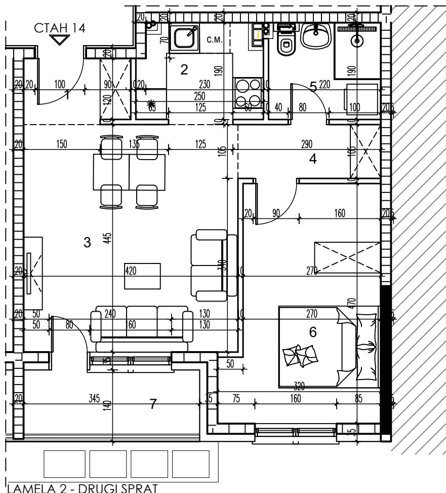
OSNOVA
