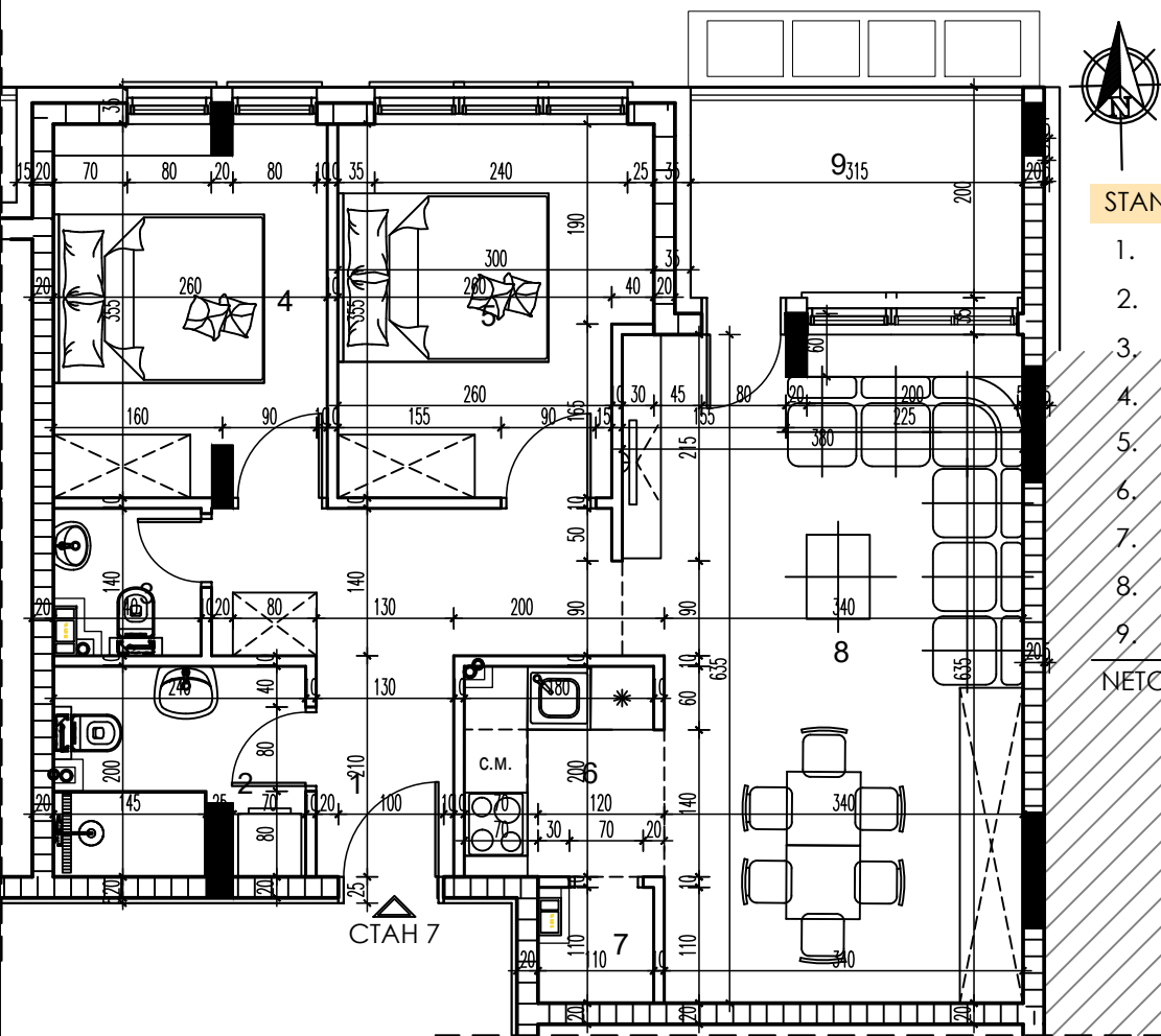
LAMELA 2 - PRVI SPRAT
