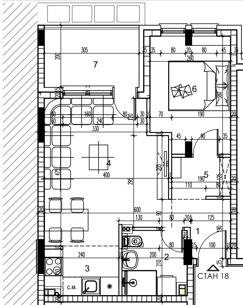
LAMELA 2 - TREĆI SPRAT
