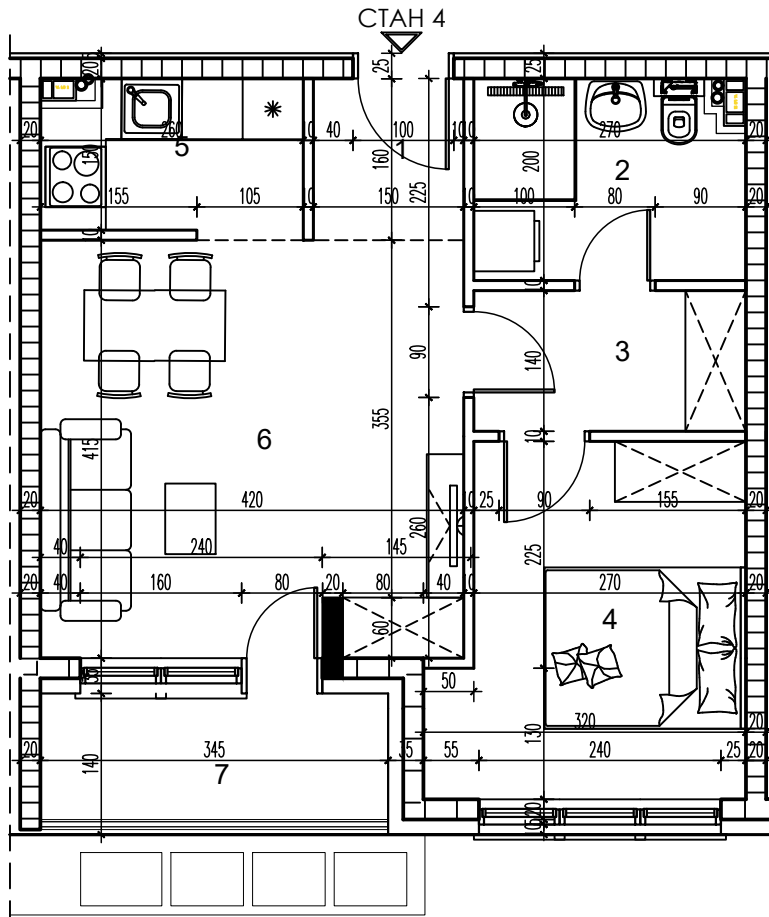
LAMELA 2 - PRVI SPRAT
