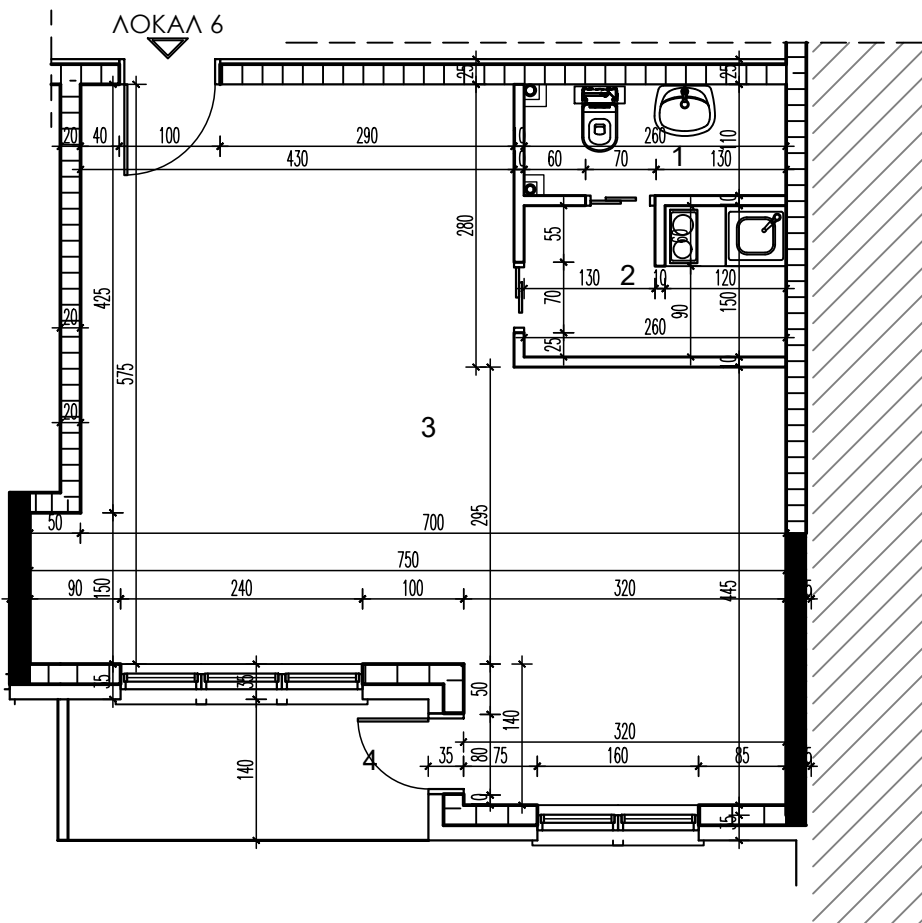
LAMELA 2 - PRIZEMLJE
