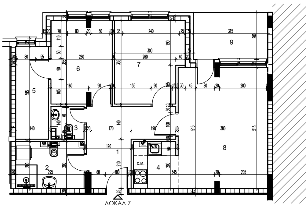
LOKAL 7
