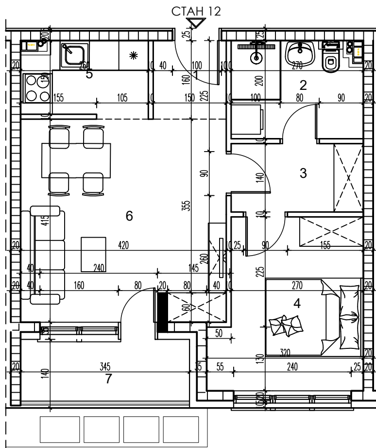
LAMELA 2 - DRUGI SPRAT
