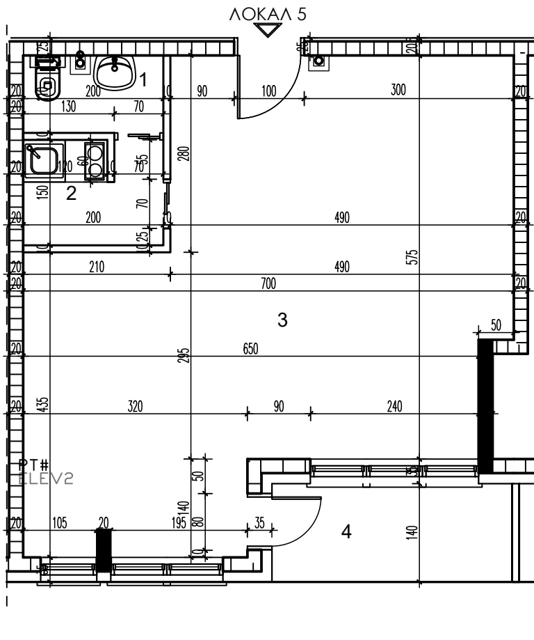
LAMELA 2 - PRIZEMLJE
