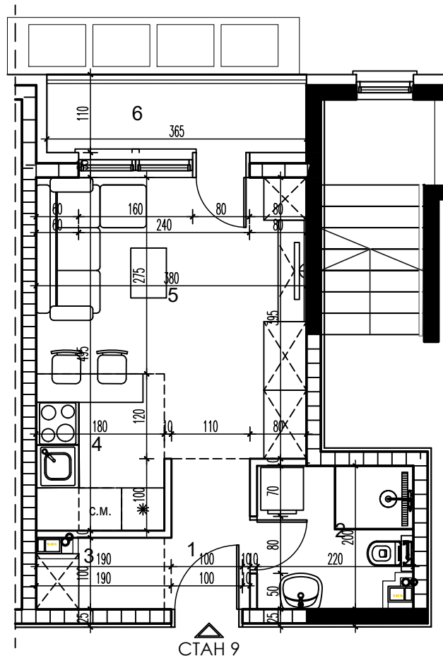
LAMELA 2 - DRUGI SPRAT
