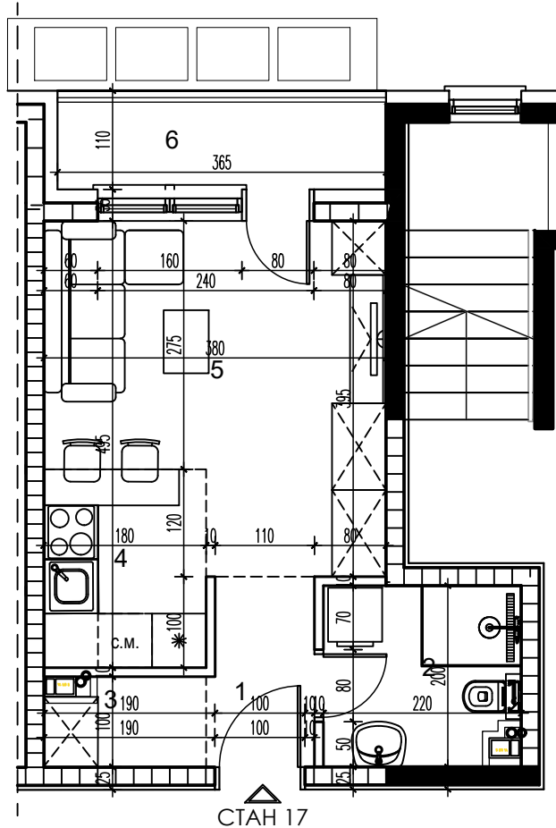
LAMELA 2 - TREĆI SPRAT
