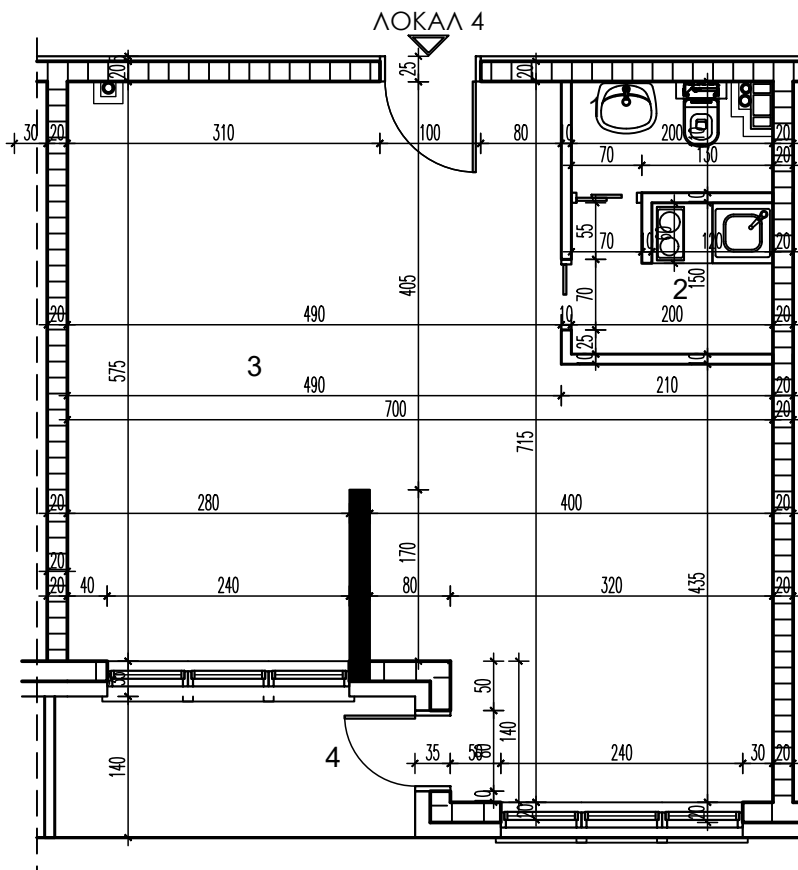
LAMELA 2 - PRIZEMLJE
