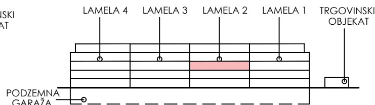
FASADA
