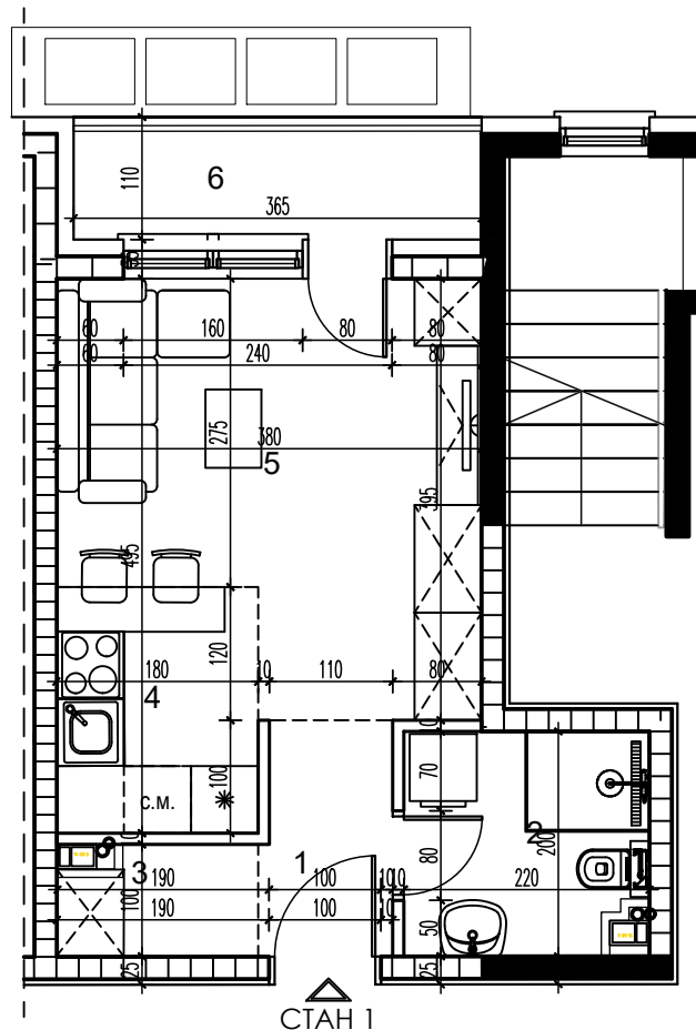
LAMELA 2 - PRVI SPRAT
