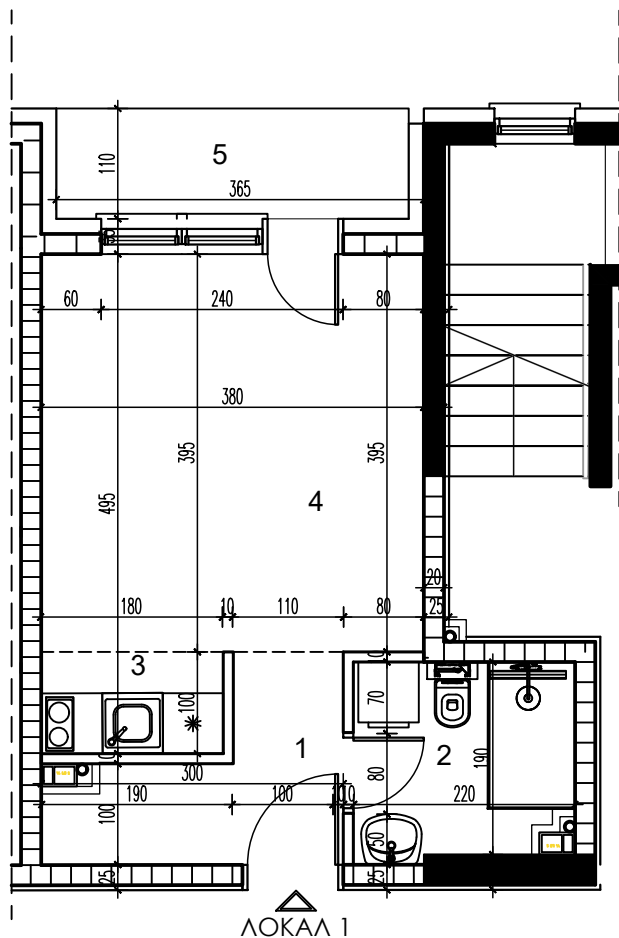
LAMELA 2 - PRIZEMLJE
